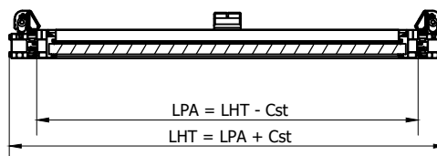
B-B ( 1:10 )
