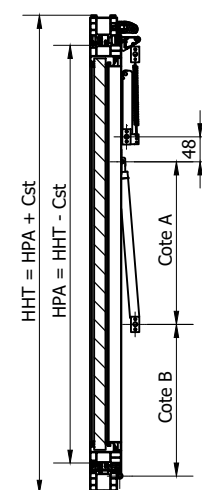
A-A ( 1:10 )
